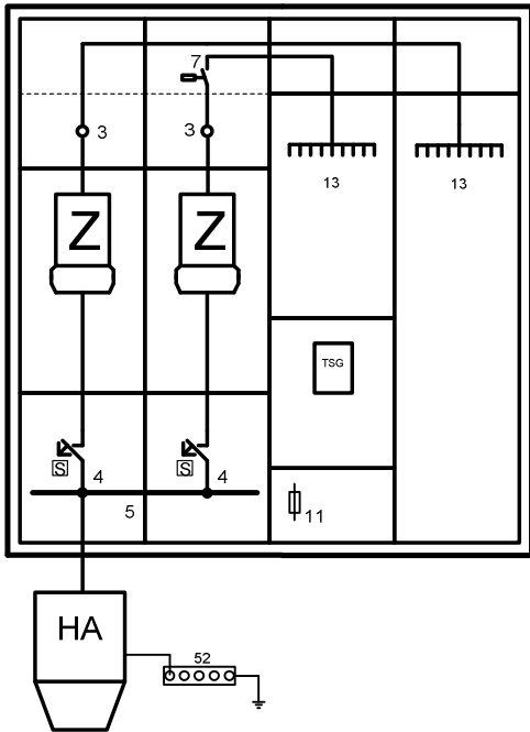
P 1.05 Einkundenanlage mit Freigabe- steuerung (Einfamilienhaus) TSG extern
