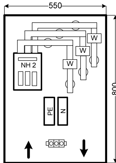
A 2.05 Wandlerschrank 800 x 550 mm (Primärnennstrom max.: 250 A)
